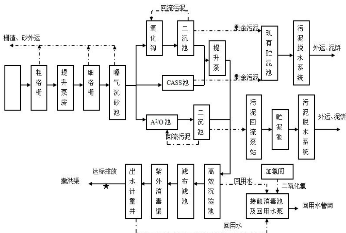
图 2-1 星沙污水处理厂处理工艺流程图
