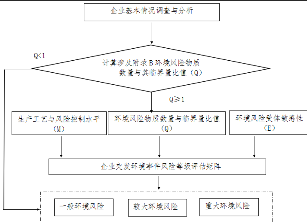
图 4-1 星沙污水处理厂突发环境事件风险等级划分流程示意图
